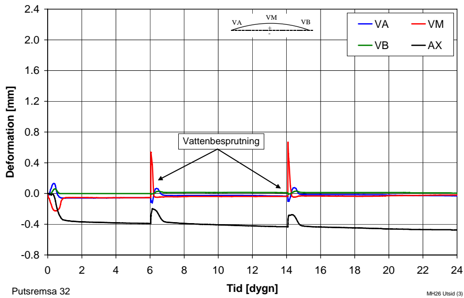
Figur 16 Deformationer hos 10 mm enkelarmerad putsremsa, icke förankrad utan isolering. Stålnät nära utsidan. Putstremsa 32.
