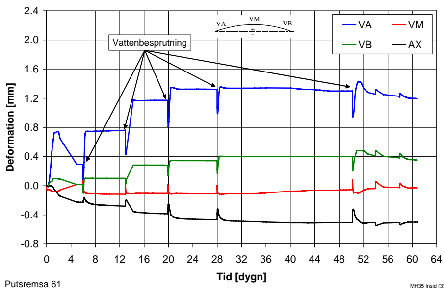
Figur 25 Deformationer hos tvåskiktputs. 10 mm armerat B-bruk + 10 mm icke armerat C-bruk, kortidskonditionering. Icke förankrad utan isolering. Stålnät i mitten av B-bruk. Putsremsa 61.
