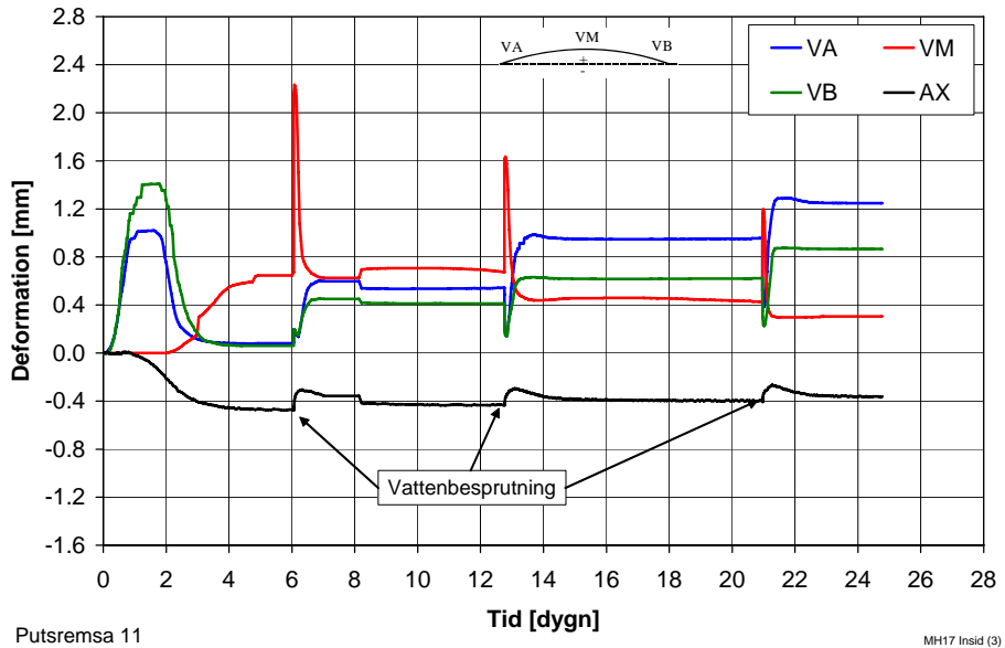
Figur 7 Deformationer hos 10 mm enkelarmerad putsrensa, icke förankrad. Stålnät nära insidan. Puttsrensa 11.
