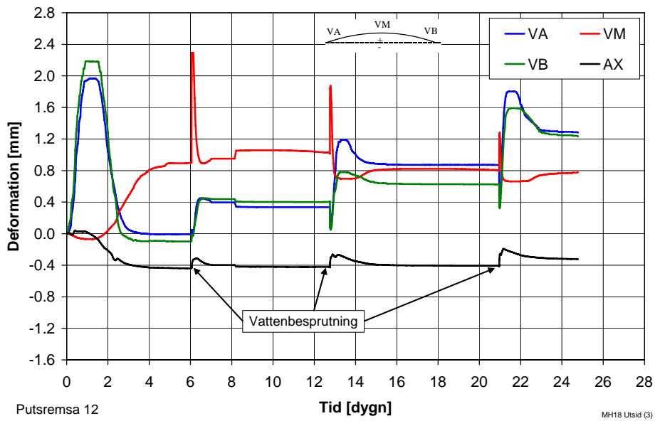
Figur 8 Deformationer hos 10 mm enkelarmerad putsrensa, icke förankrad. Stålnät nära utsidan. Puttsrensa 12.
