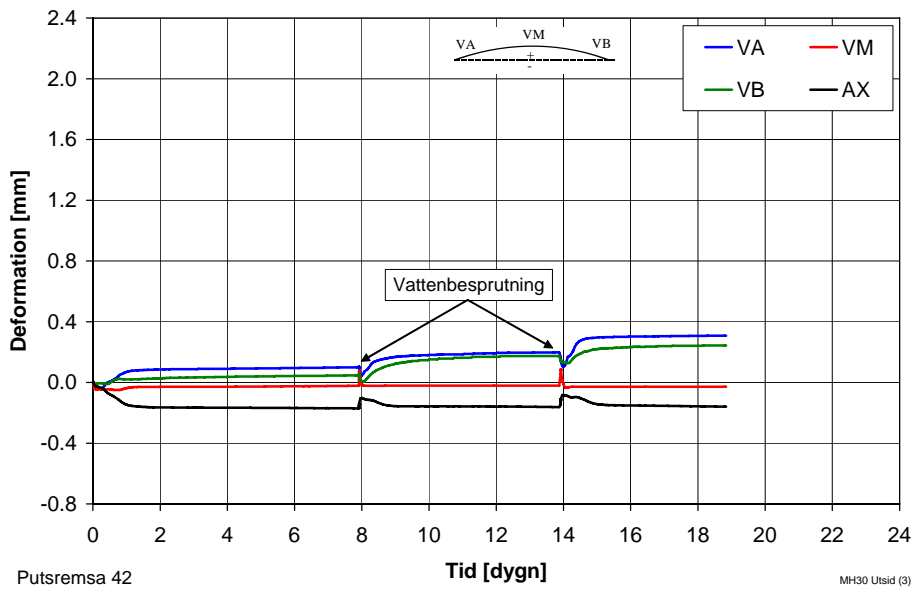
Figur 20 Deformationer hos 10 mm enkelarmerad putsremsa, icke förankrad utan isolering. Stålnät nära utsidan. C-Bruk. Putstremsa 42.
