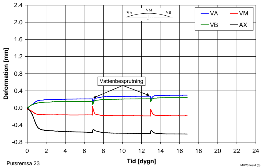
Figur 13 Deformationer hos 10 mm enkelarmerad putsremsa, förankrad med isolering. Stålnät nära insidan. Puttsremsa 23.
