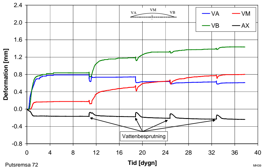
Figur 30 Deformationer hos 10 mm armerad putsremsa. C-bruk SERPO 136, 7 dygnshärdning, Icke förankrad utan isolering. Stålnät nära insidan. Putstremsa 72.
