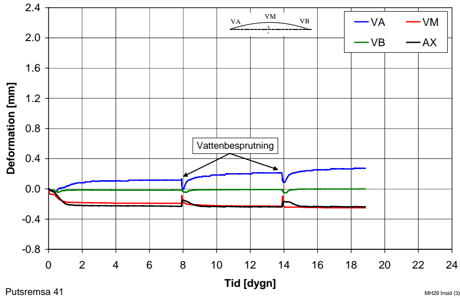
Figur 19 Deformationer hos 10 mm enkelarmerad putsremsa, icke förankrad utan isolering. Stålnät nära insidan. C-Bruk. Putstremsa 41.
