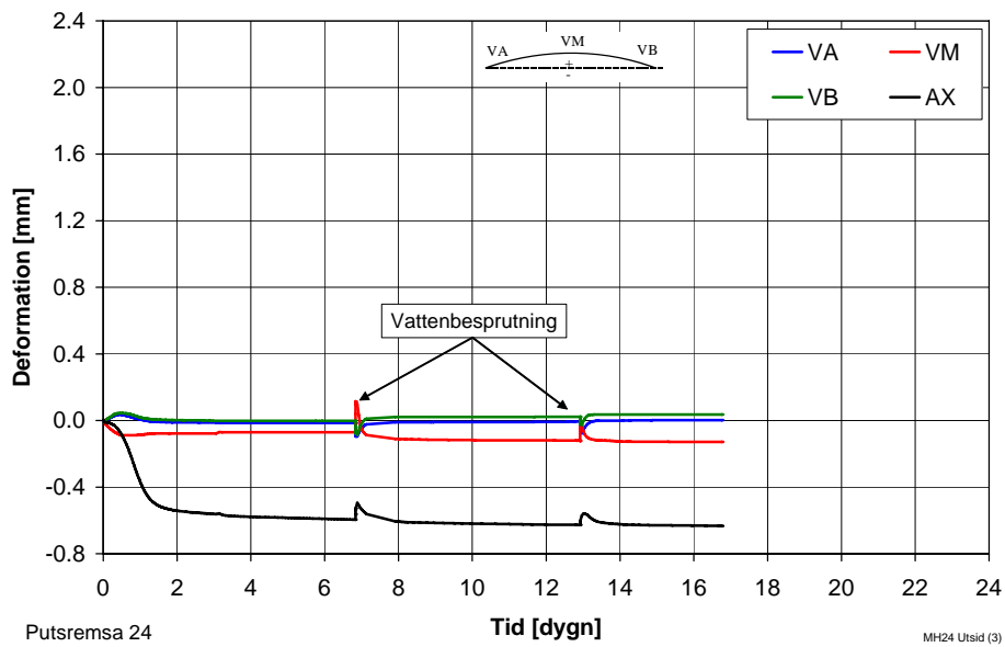
Figur 14 Deformationer hos 10 mm enkelarmerad putsremsa, förankrad med isolering. Stålnät nära utsidan. Puttsremsa 24.
