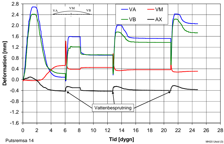
Figur 10 Deformationer hos 10 mm enkelarmerad putsrensa, icke förankrad. Glasfibernät nära utsidan. Puttsrensa 14.
