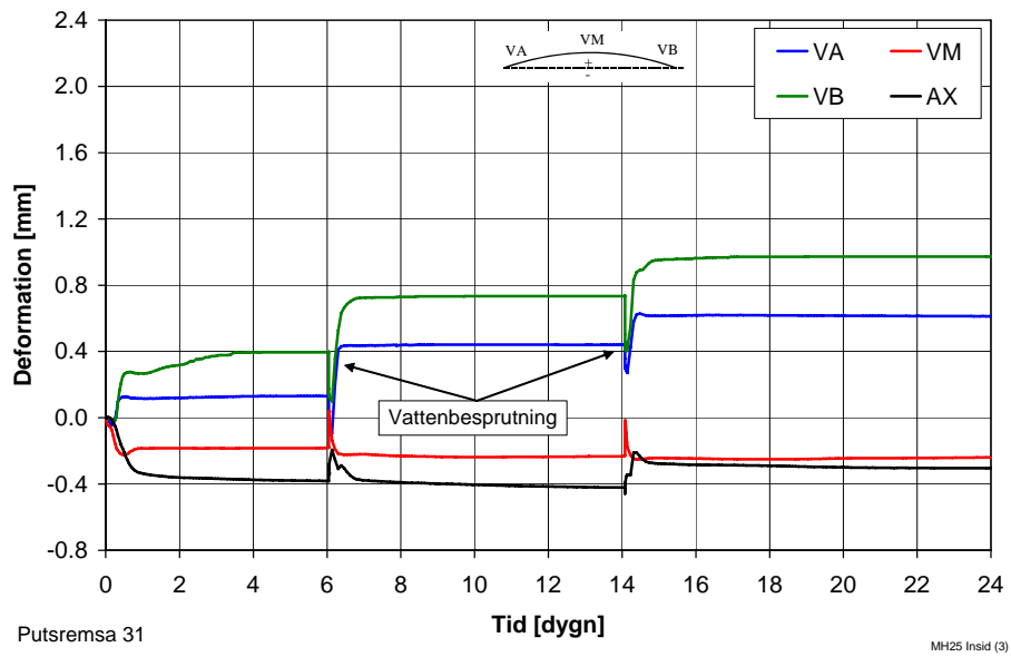
Figur 15 Deformationer hos 10 mm enkelarmerad putsremsa, icke förankrad utan isolering. Stålnät nära insidan. Putstremsa 31.
