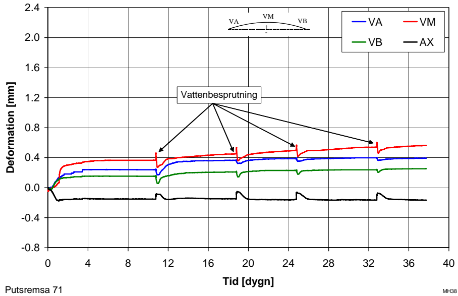
Figur 29 Deformationer hos 10 mm armerad putsremsa. C-bruk SERPO 136, 3 dygnshärdning, Icke förankrad utan isolering. Stålnät nära insidan. Putstremsa 71.
