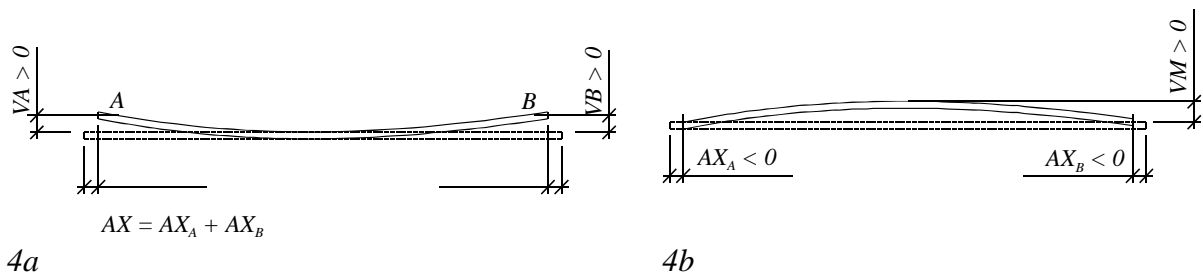
Figur 4 Axiell deformation ( AX ) och deformationer vinkelräta mot putsremsans längdaxel ( VA , VB och VM ).
