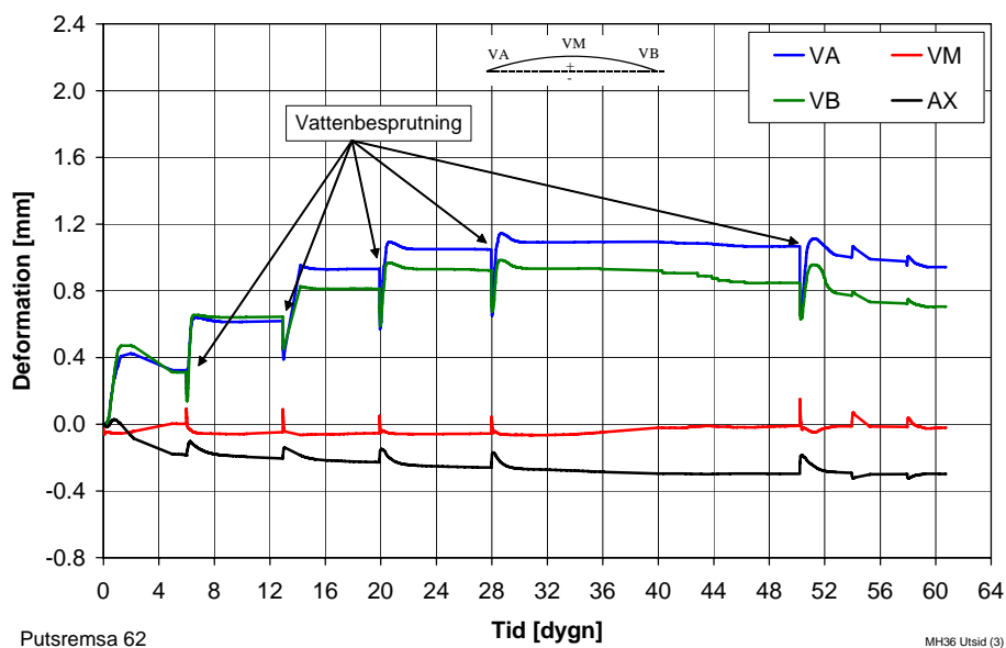
Figur 26 Deformationer hos tvåskiktputs. 10 mm armerat B-bruk + 10 mm icke armerat C-bruk, långtidskonditionering. Icke förankrad utan isolering. Stålnät i mitten av B-bruk. Putsremsa 62.
